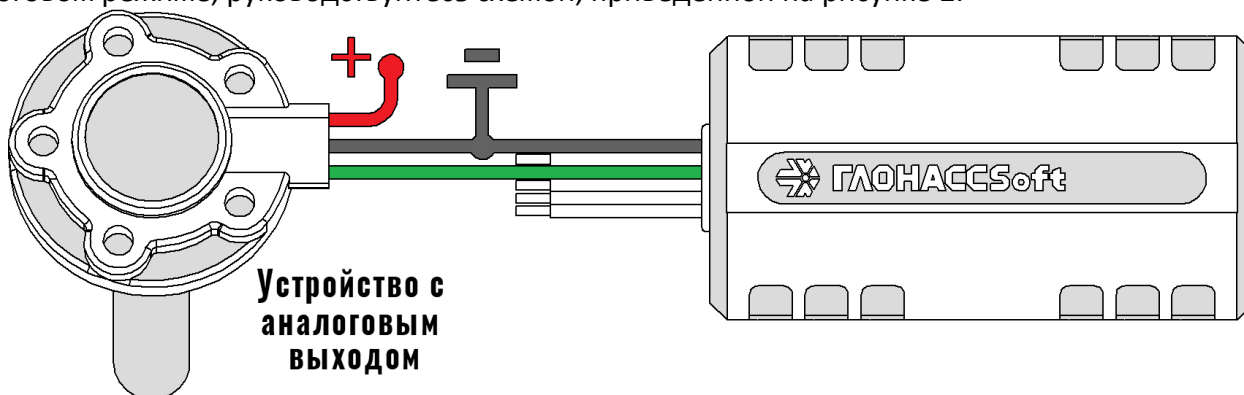
Рисунок 2 – Подключение ДУТ в аналоговом режиме.
