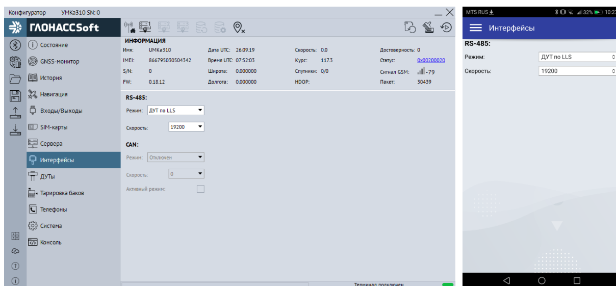
Рисунок 3 – Вкладка «Интерфейсы».
